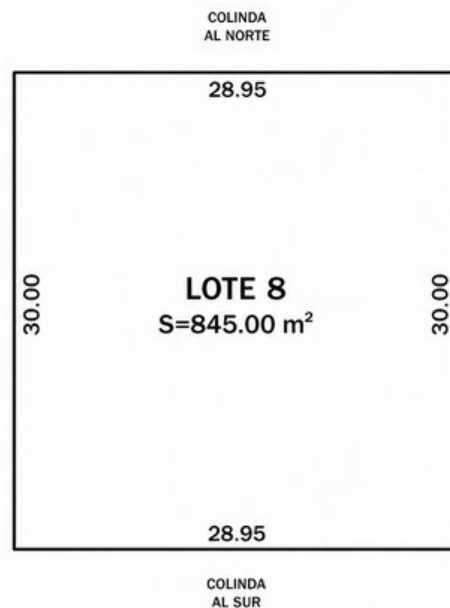
PLANO TOPOGRAFICO
