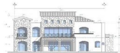
FACHADA SUR
